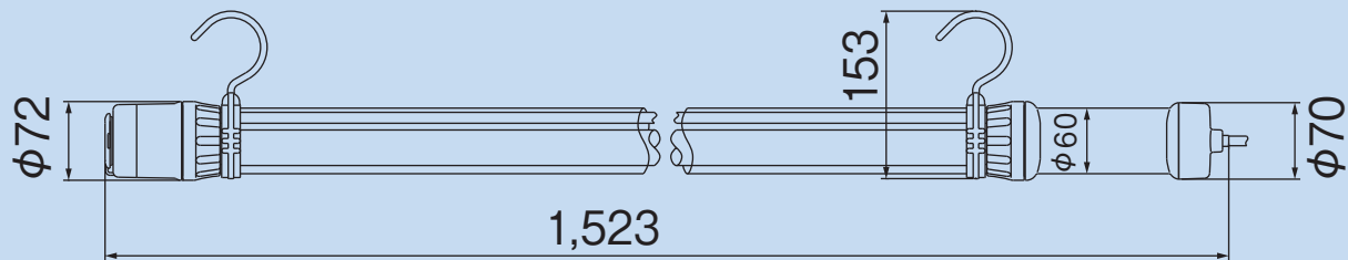
FXW型
