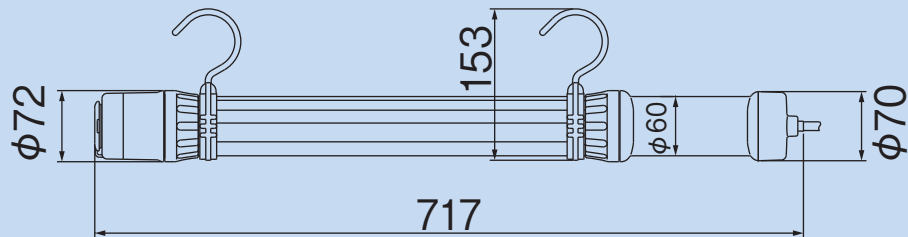
FJW型
